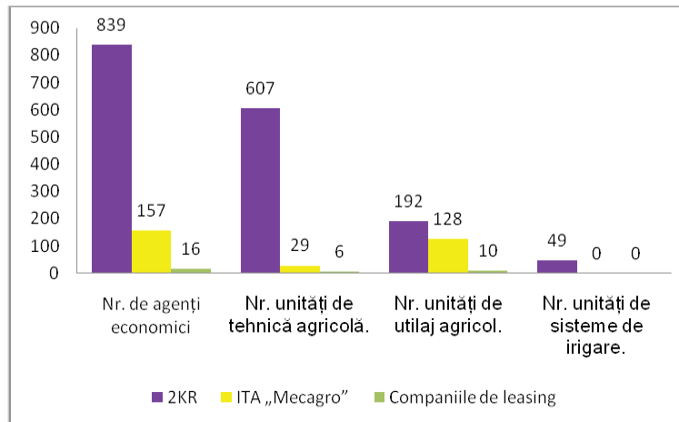
Figura 5. Tehnica agricolă procurată în anul 2014 prin intermediul 2KR, ITA „Mecagro” și a companiilor de leasing.
