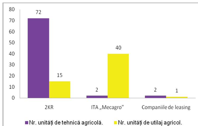
Figura 4. Tehnica agricolă procurată în anul 2015 prin intermediul 2KR, ITA „Mecagro” și a companiilor de leasing.
